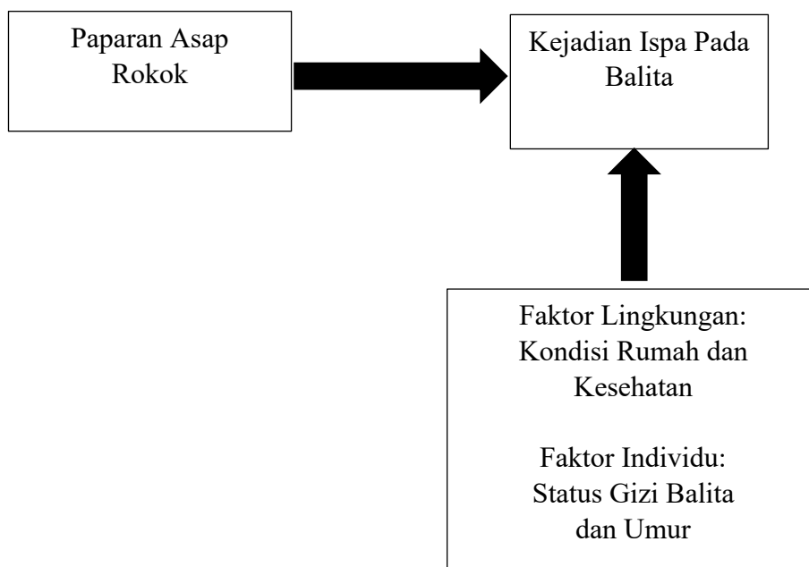
Gambar 1 Kerangka konsep
