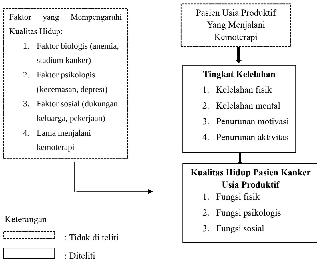
Gambar 1 Kerangka Konsep
