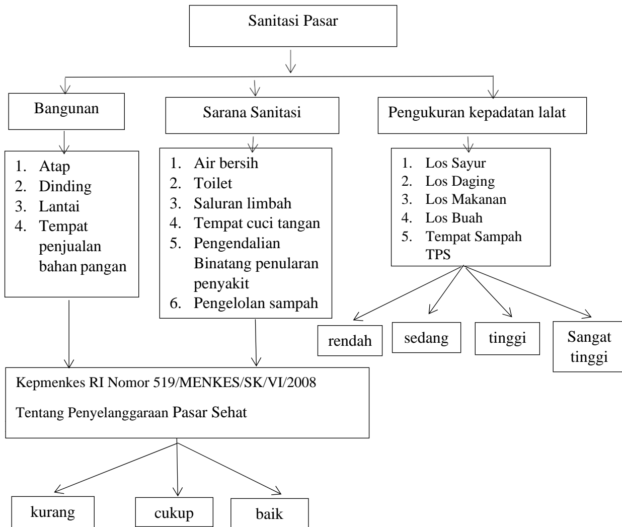
Gambar 2 Kerangka Konsep
