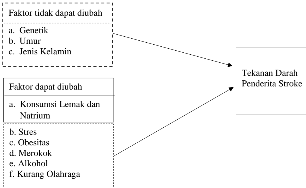
Gambar 1 Kerangka Konsep
