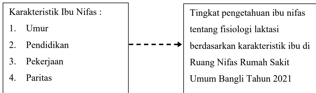
Gambar 1. Kerangka konsep
