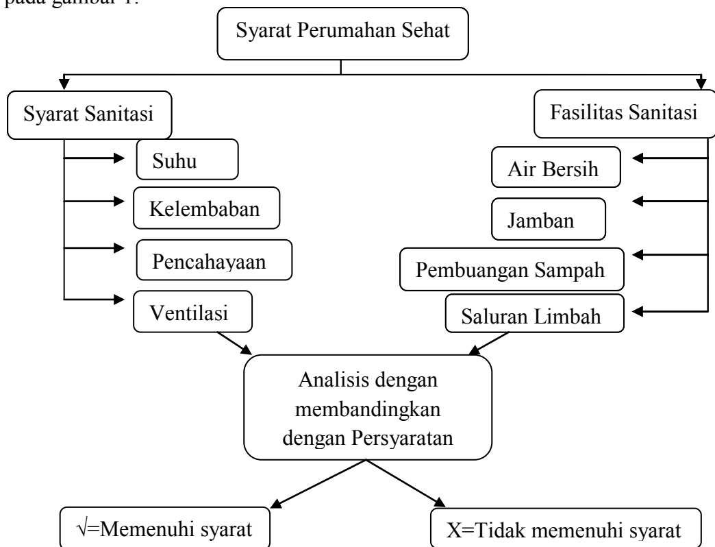
Gambar 1 Kerangka Konsep
