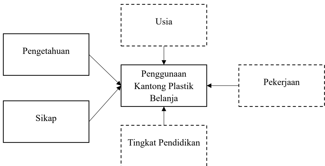
Gambar 1 Kerangka Konsep
