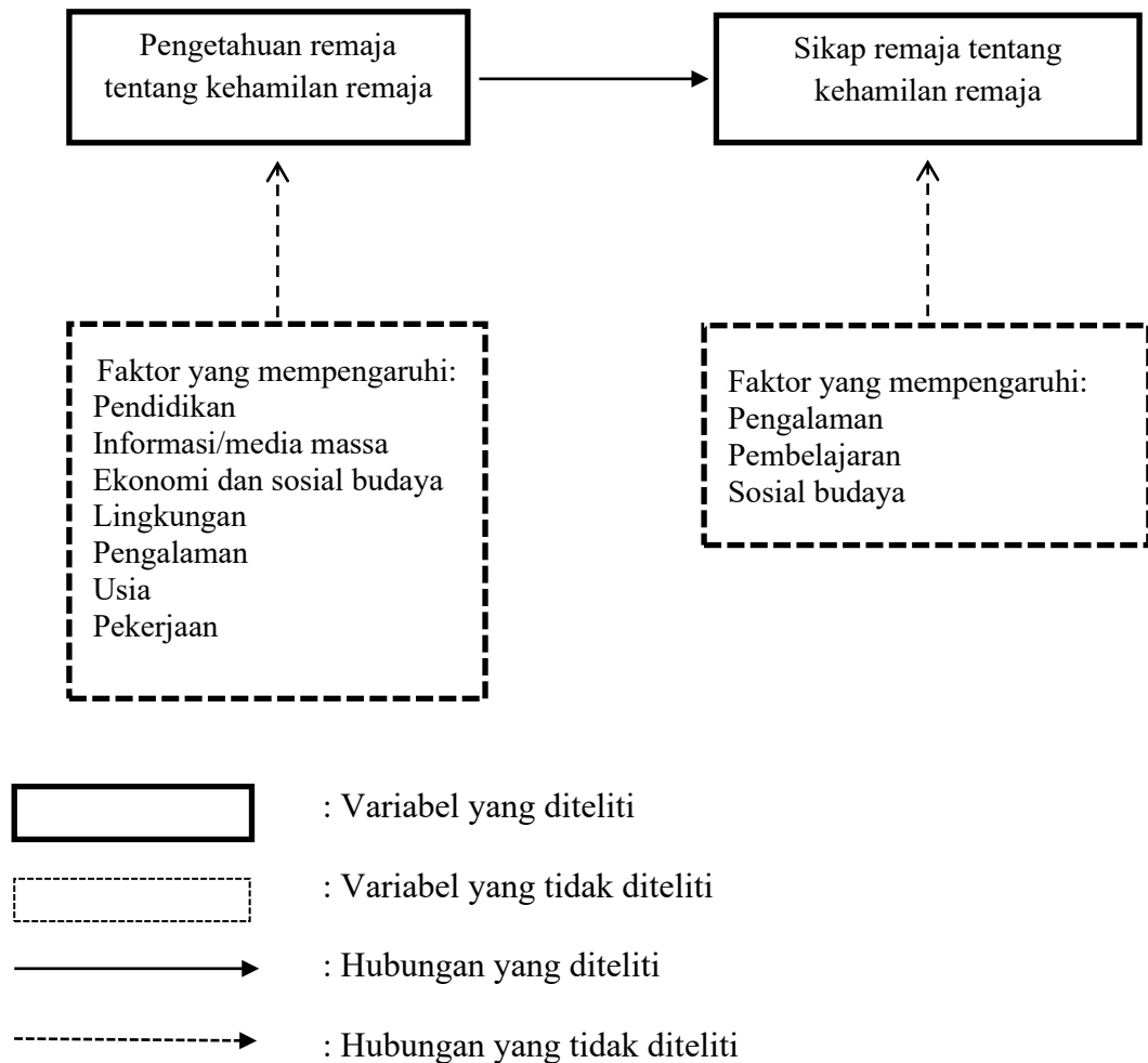
Gambar 1. Kerangka Konsep
