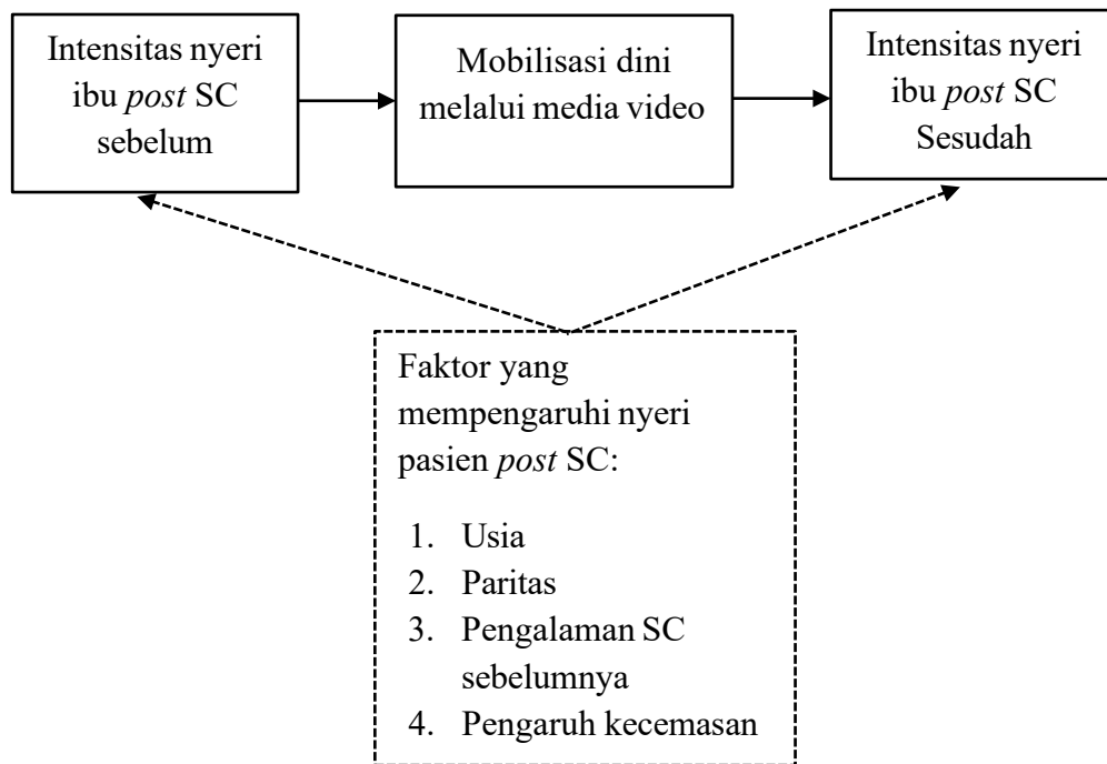
Gambar 3 Kerangka Konsep
