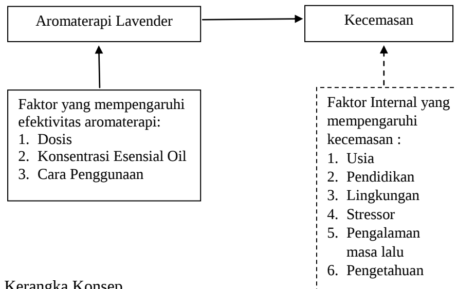
Gambar 2 Kerangka Konsep
