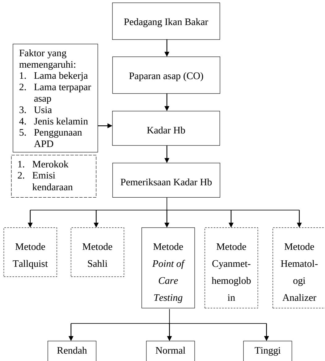
Gambar 5 Kerangka Konsep
