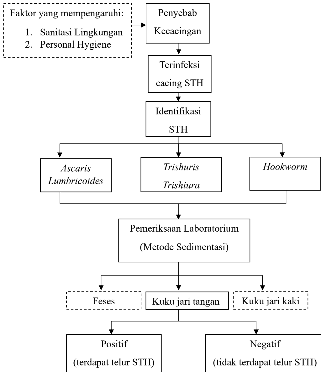
Gambar 8. Kerangka Konsep
