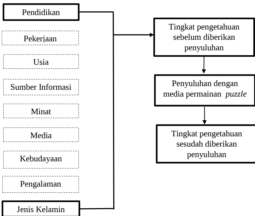
Gambar 1 Kerangka Konsep
