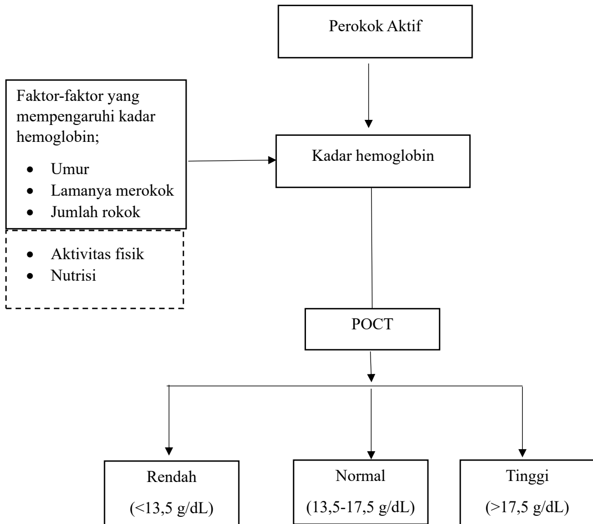
Gambar 1 Kerangka Konsep
