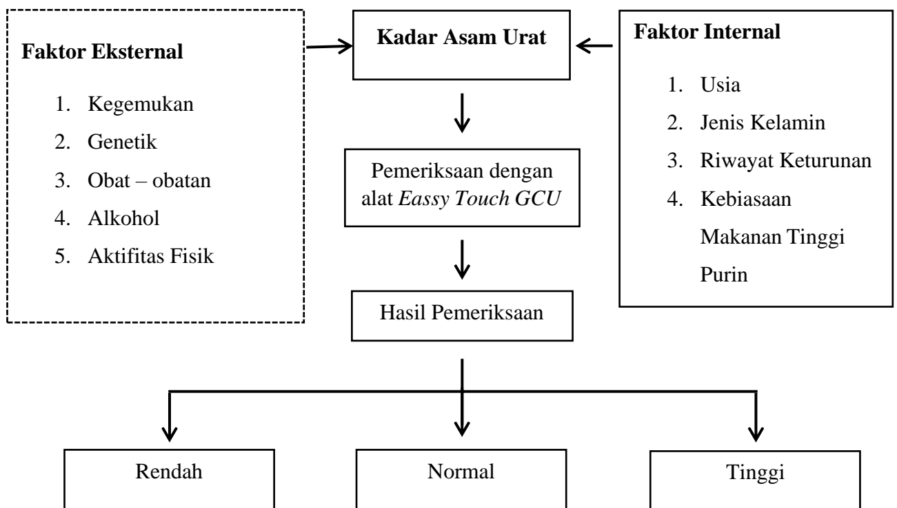
Gambar 2. Kerangka Konsep
